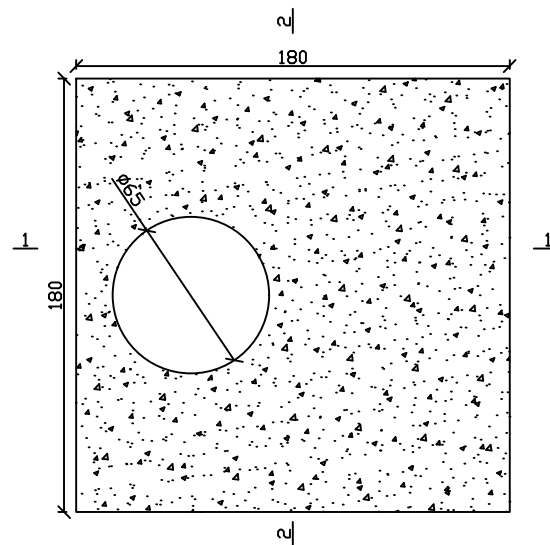
Plan placa acoperire camin
