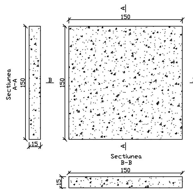
Plan radier camin
