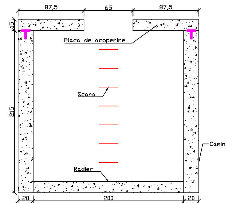
Sectiune camin 2-2
