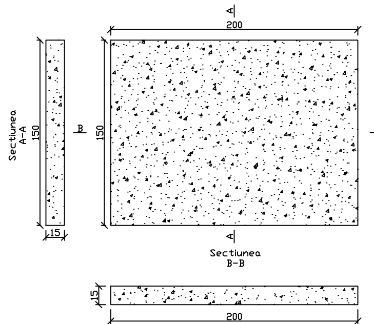
Plan radier camin
