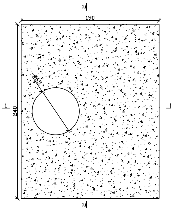
Plan placa acoperire camin
