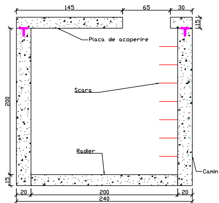
Sectiune camin 1-1
