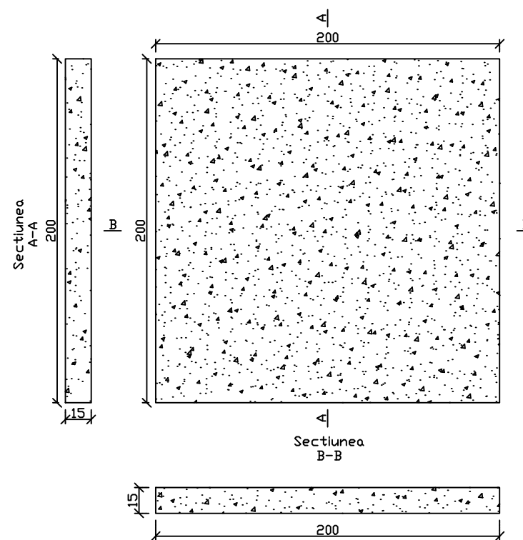
Plan radier camin
