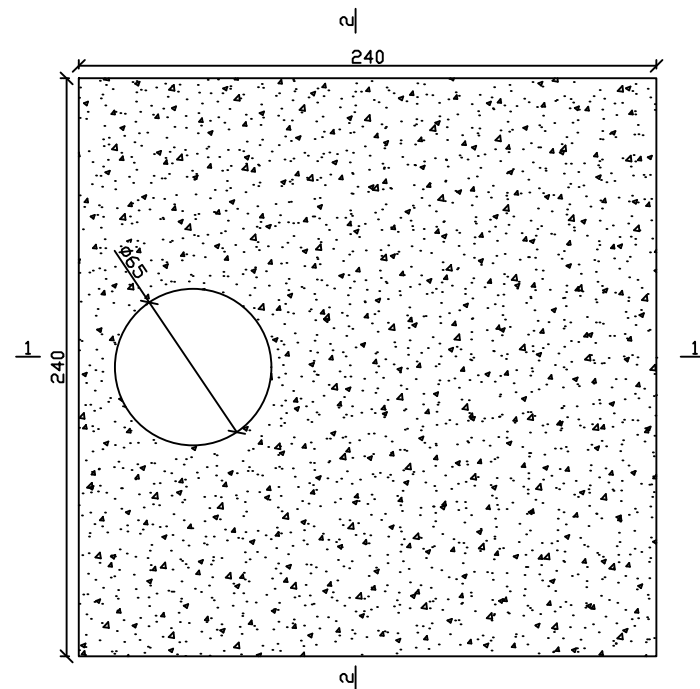
Plan placa acoperire camin
