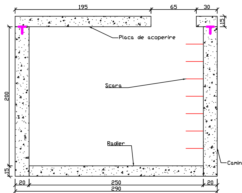
Sectiune camin 1-1
