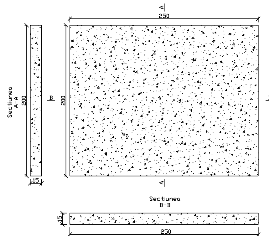
Plan radier camin
