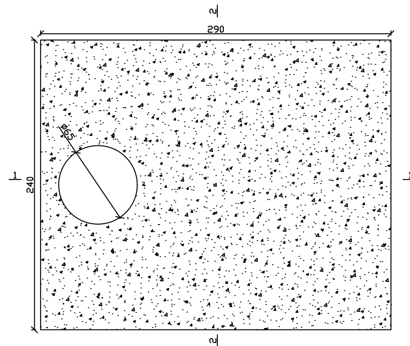
Plan placa acoperire camin
