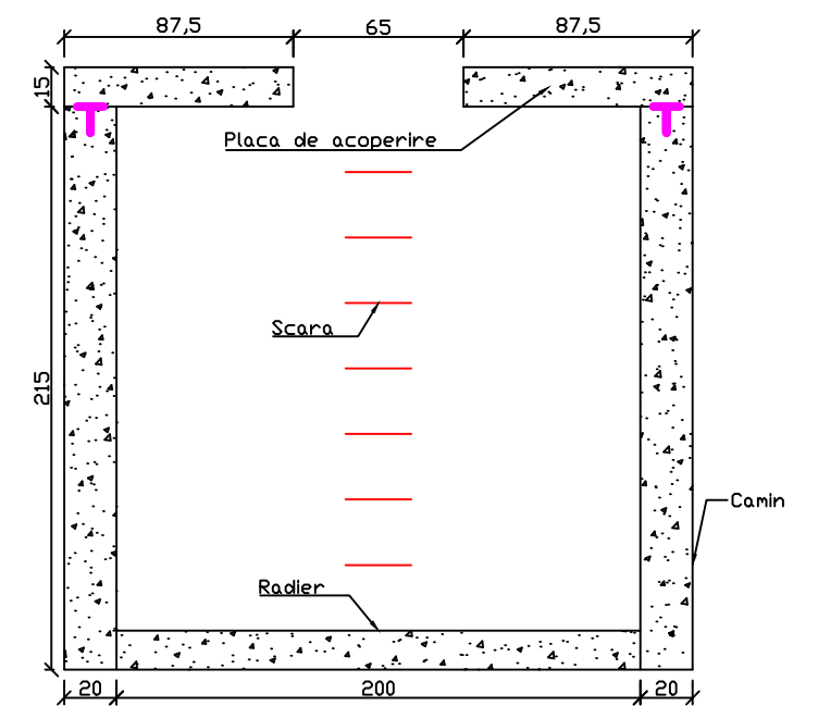
Sectiune camin 2-2
