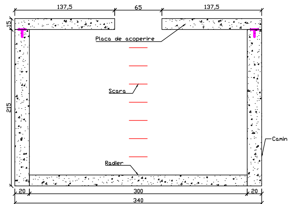
Sectiune camin 2-2
