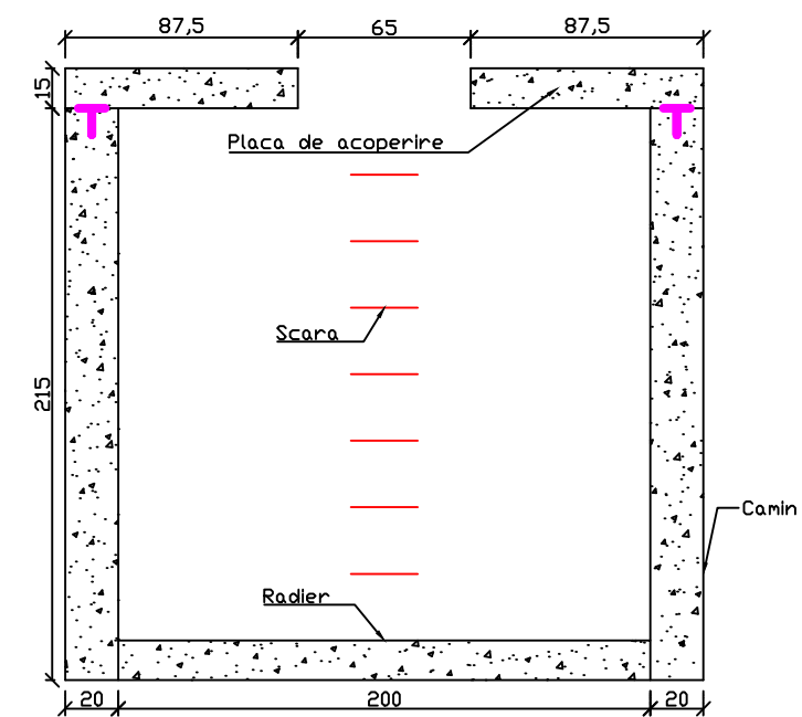
Sectiune camin 2-2
