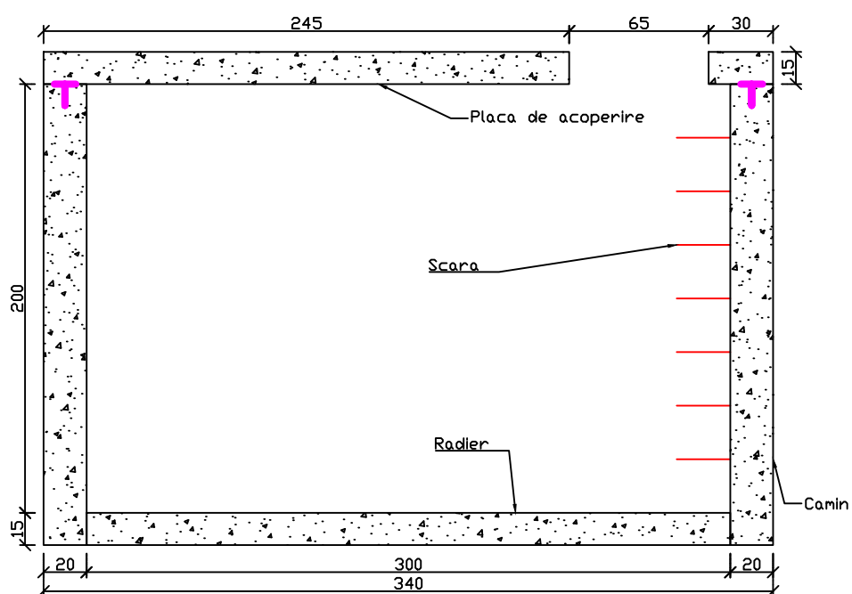
Sectiune camin 1-1
