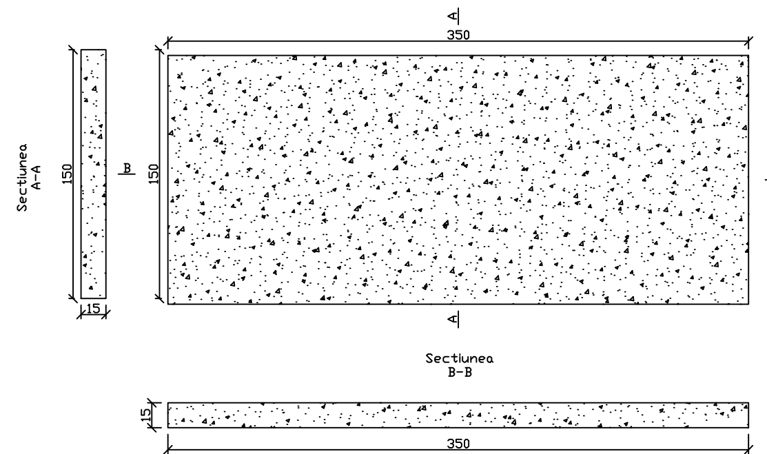
Plan radier camin
