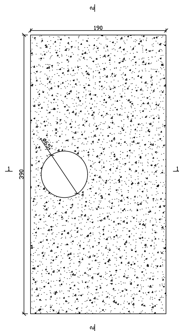
Plan placa acoperire camin
