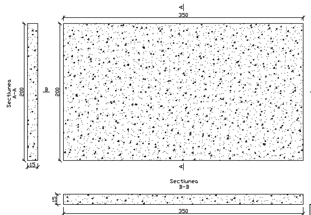
Plan radier camin
