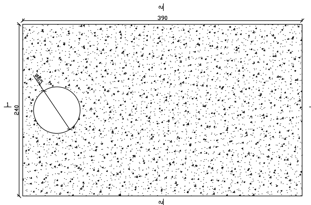
Plan placa acoperire camin
