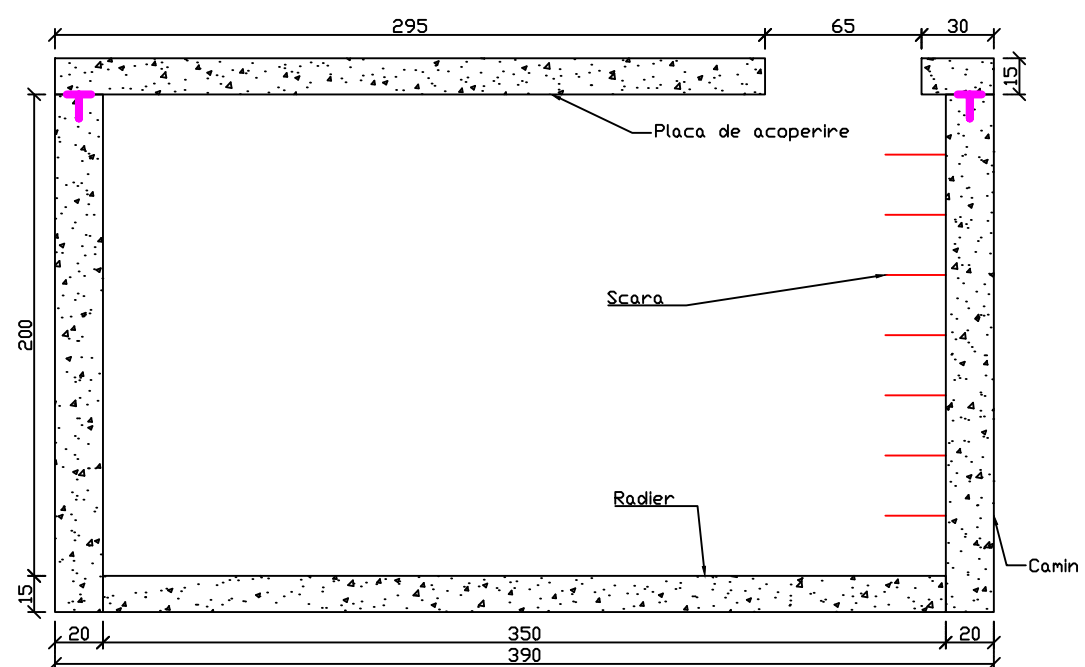
Sectiune camin 1-1
