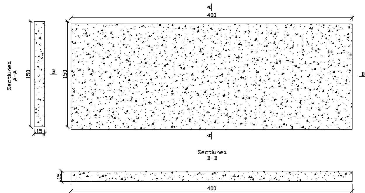
Plan radier camin
