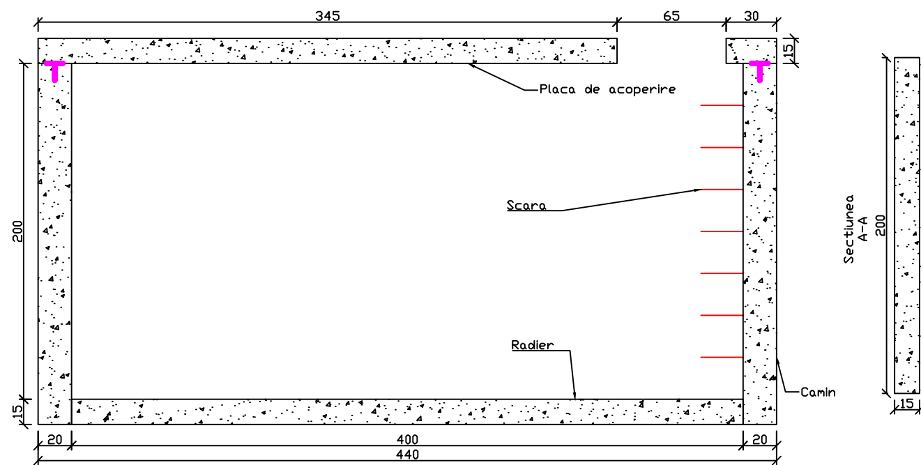
Sectiune camin 1-1
