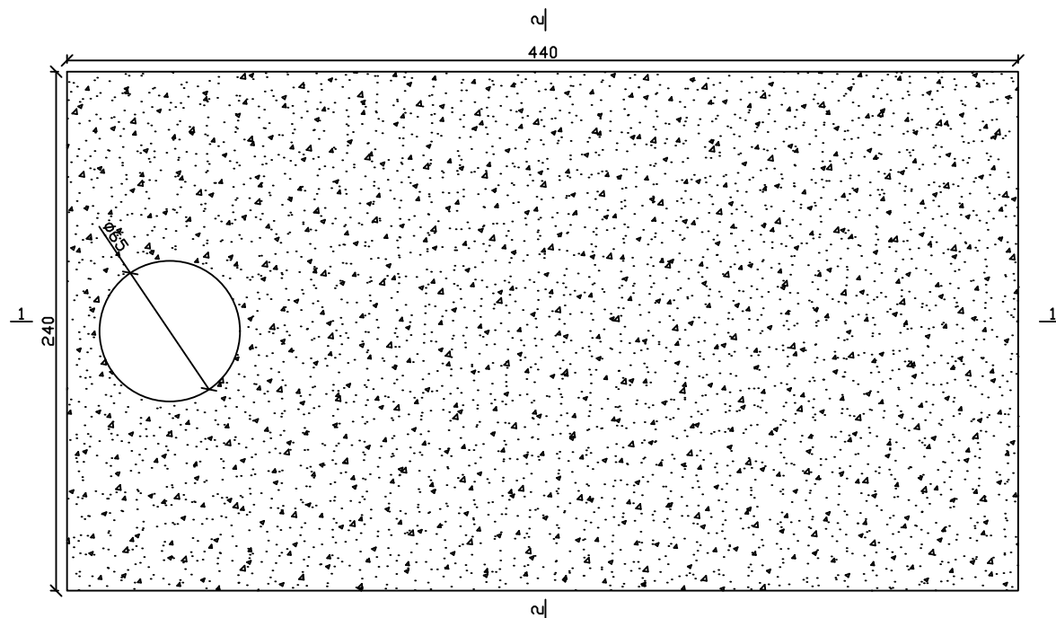
Sectiune camin 1-1
