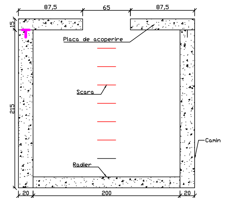
Sectiune camin 2-2
