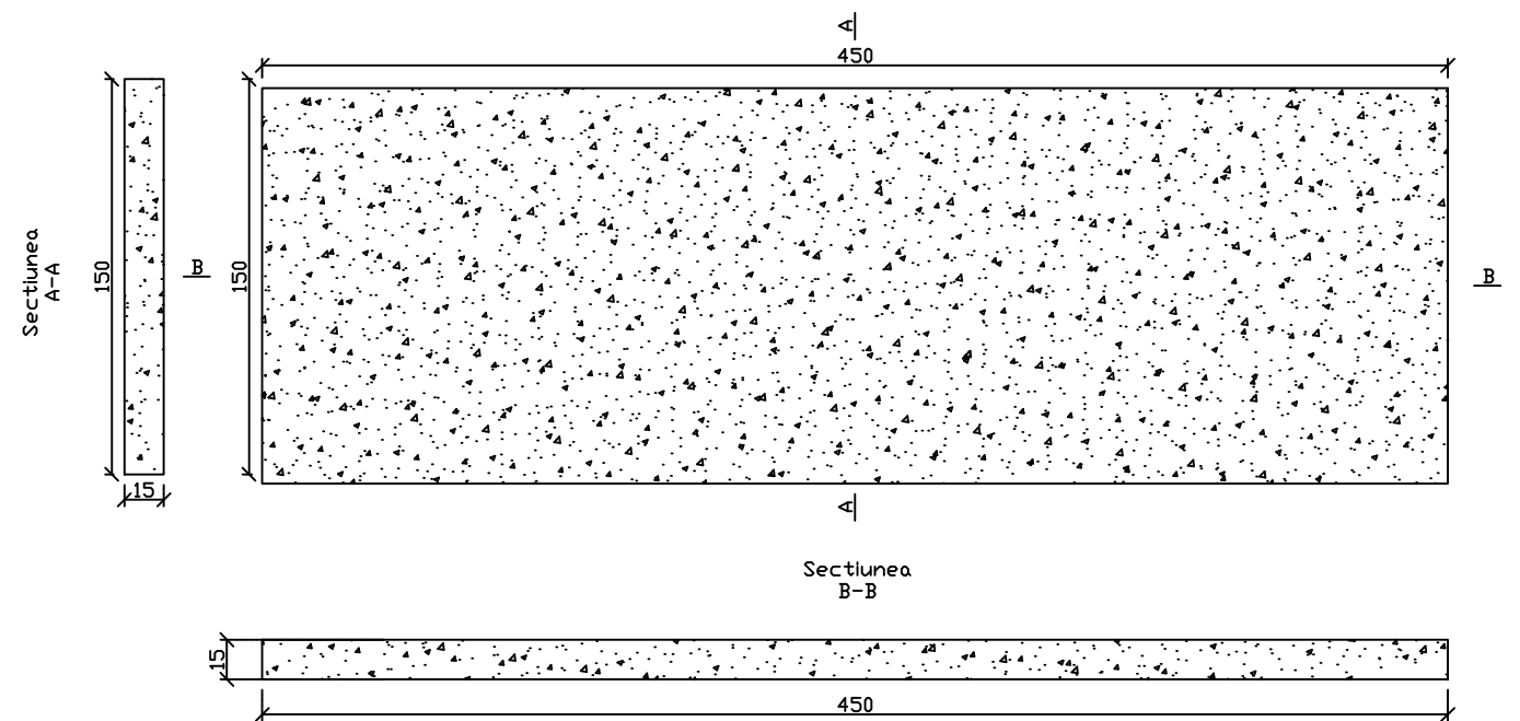
Plan radier camin
