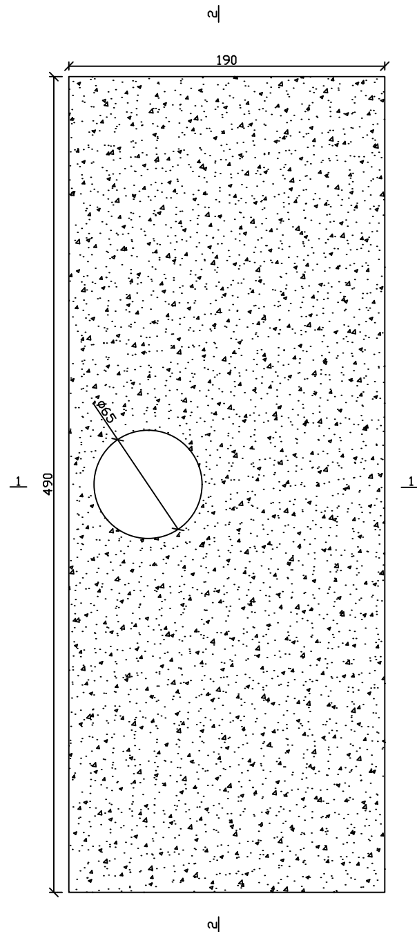
Plan placa acoperire camin
