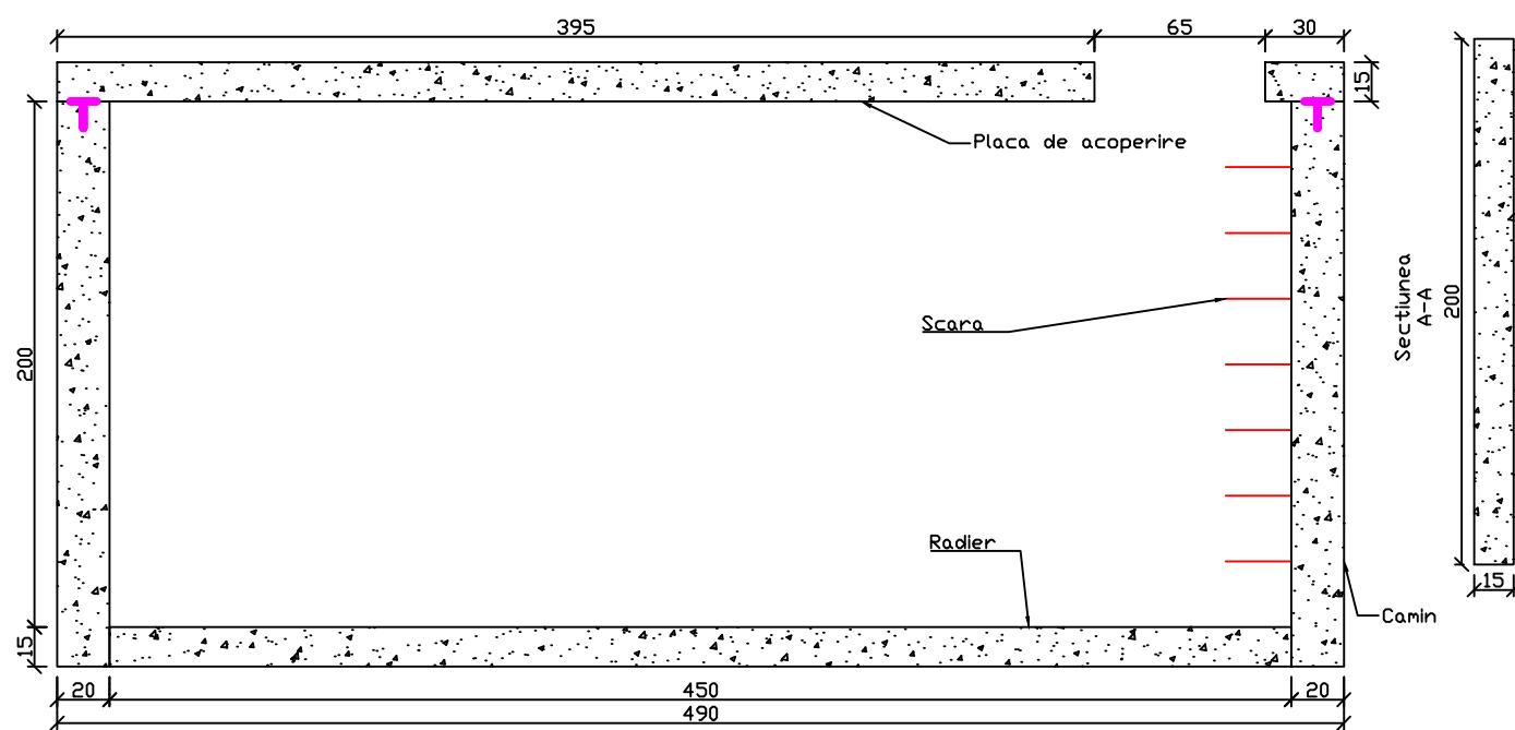
Sectiune camin 1-1
