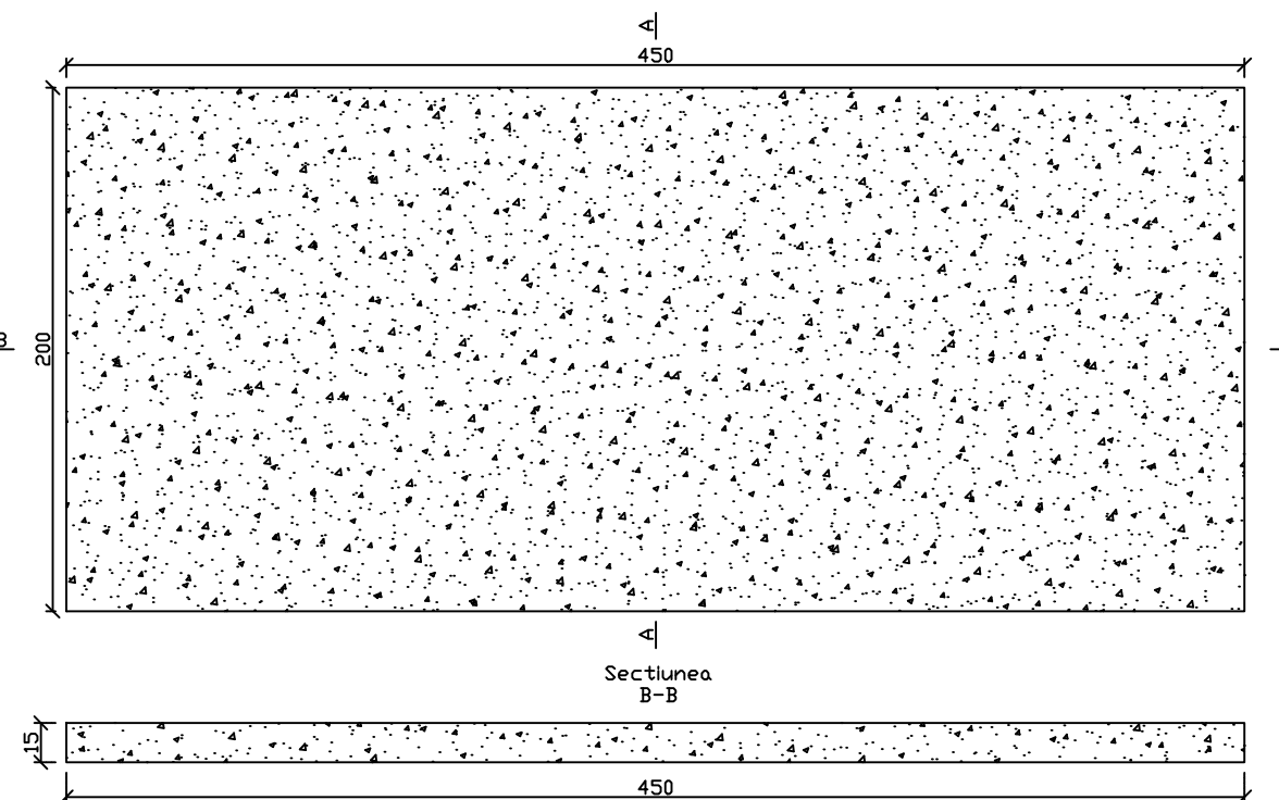
Plan radier camin
