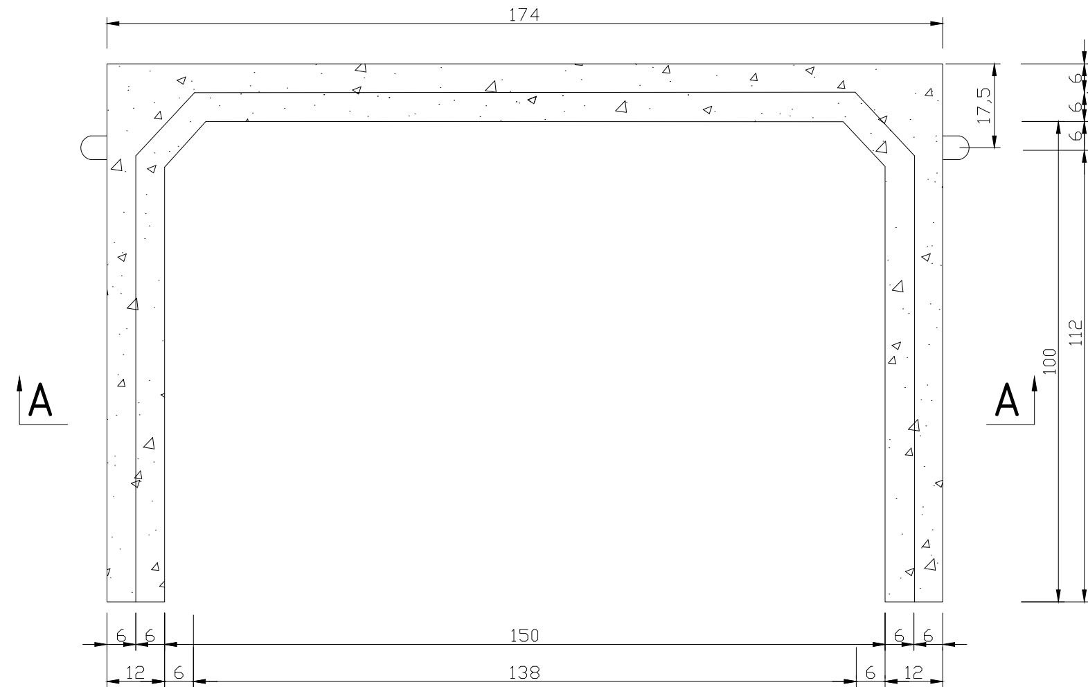
Vedere A-A
