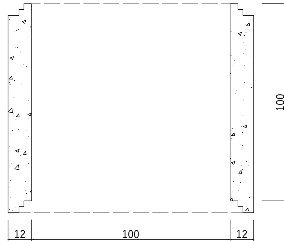
Sectiune Inel camin DN1000 H1000 G120
