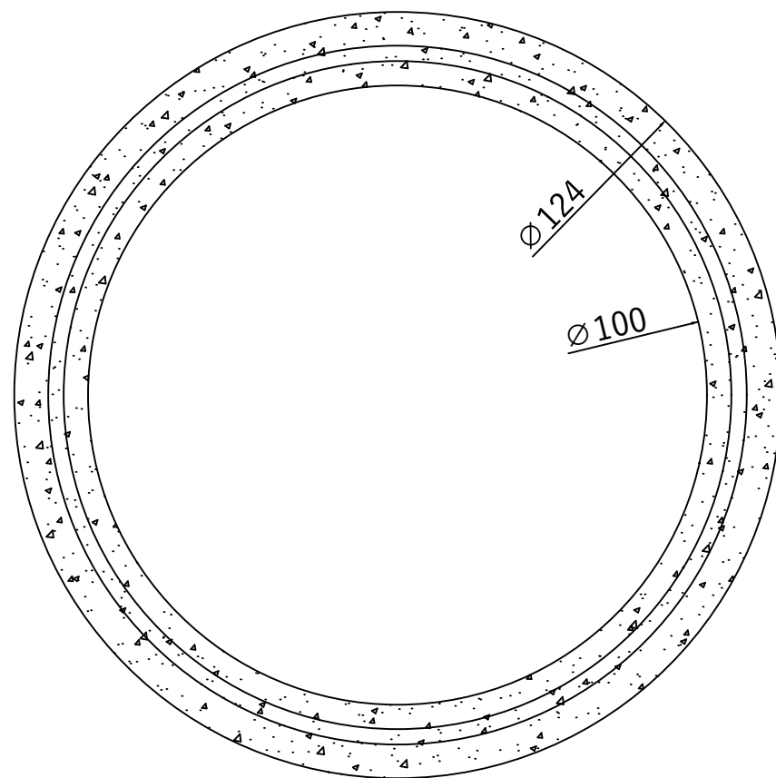
Vedere in plan Inel camin DN1000 H1000 G120
