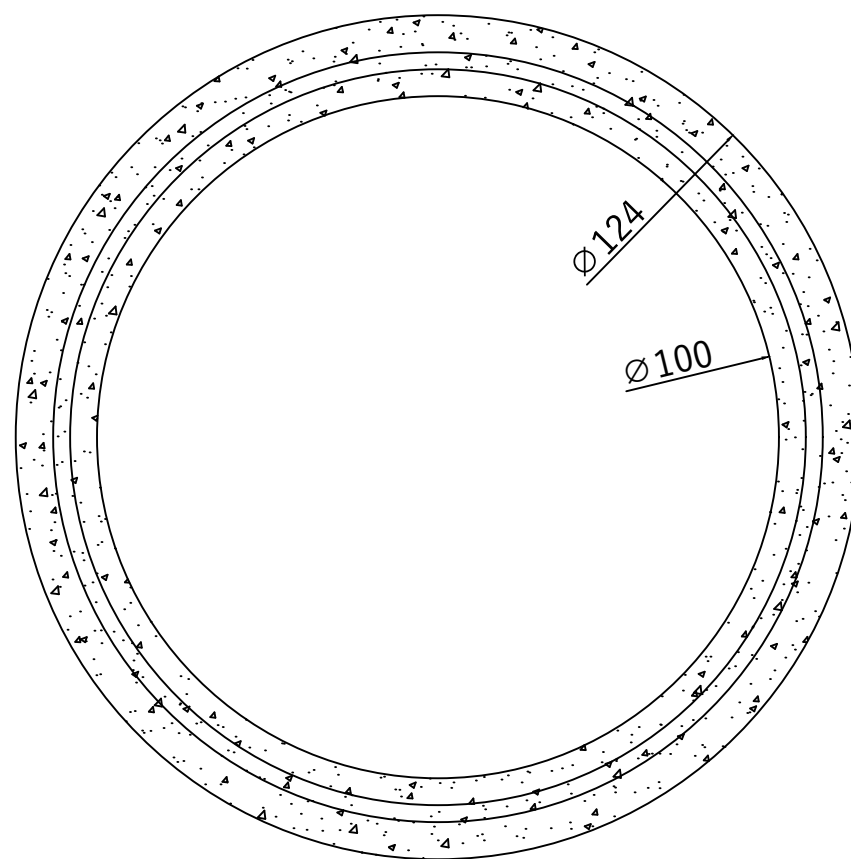
Vedere in plan Inel camin DN1000 H100 G120
