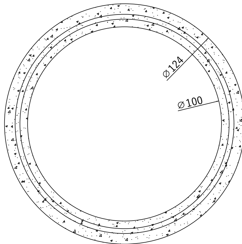
Vedere in plan Inel camin DN1000 H250 G120
