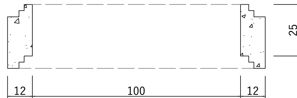
Sectiune Inel camin DN1000 H250 G120
