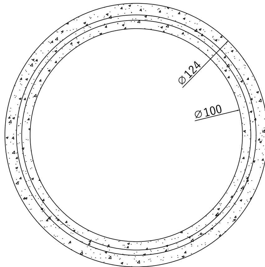
Vedere in plan Inel camin DN1000 H500 G120
