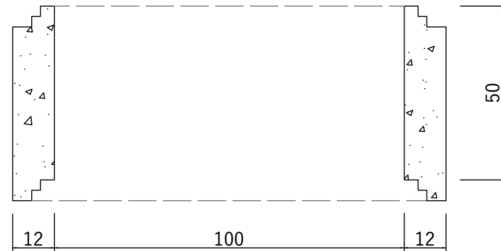
Sectiune Inel camin DN1000 H500 G120
