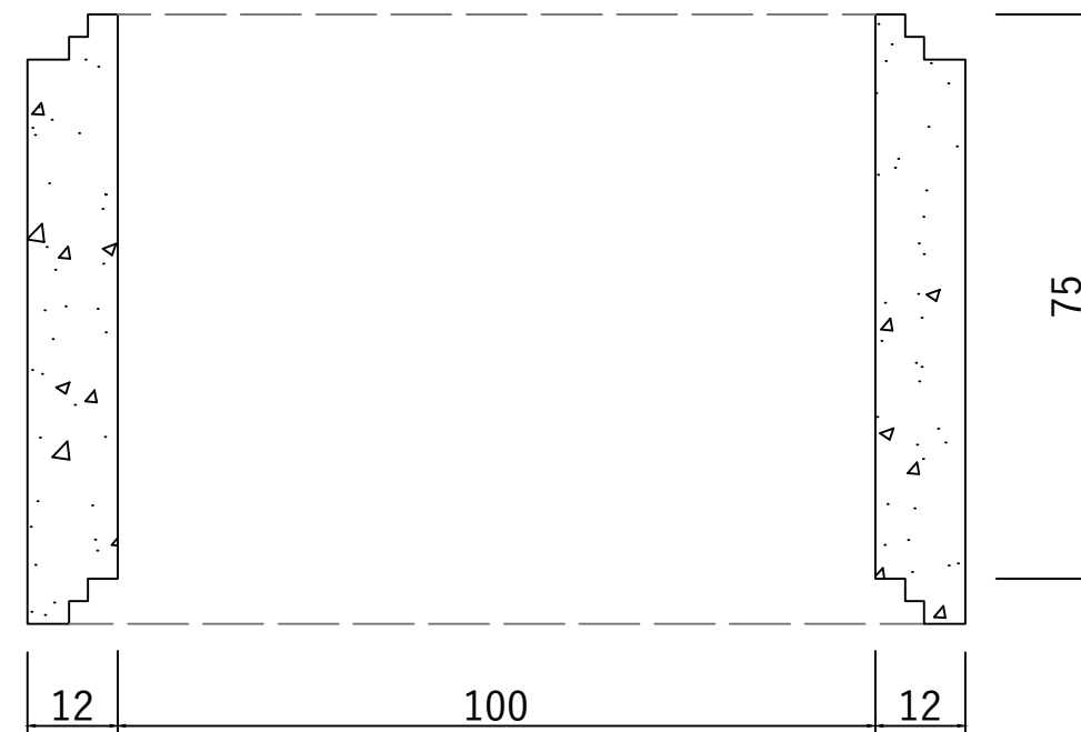
Sectiune Inel camin DN1000 H750 G120
