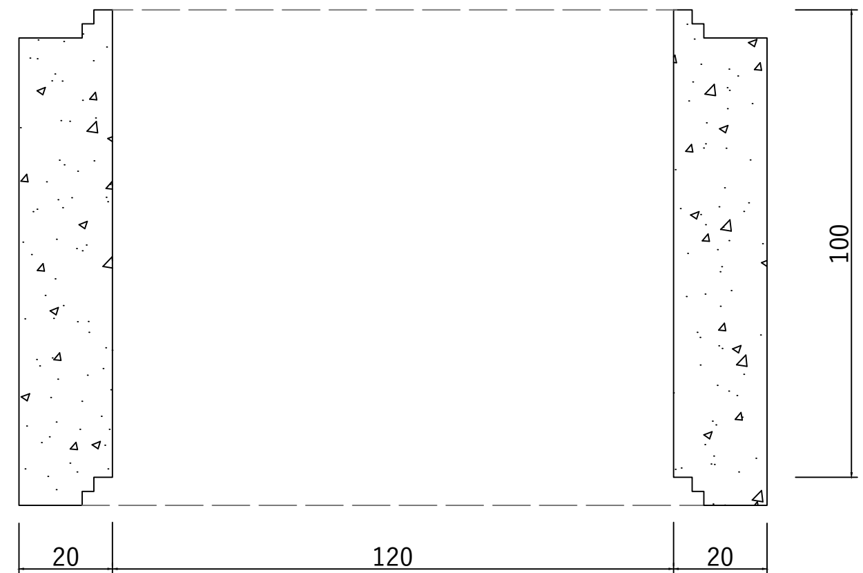
Sectiune Inel camin DN1200 H1000 G200
