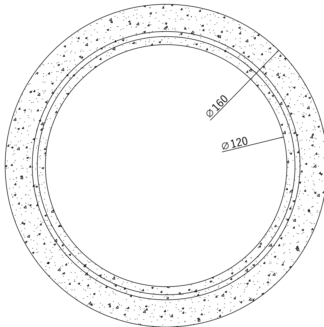
Vedere in plan Inel camin DN1200 H1000 G200
