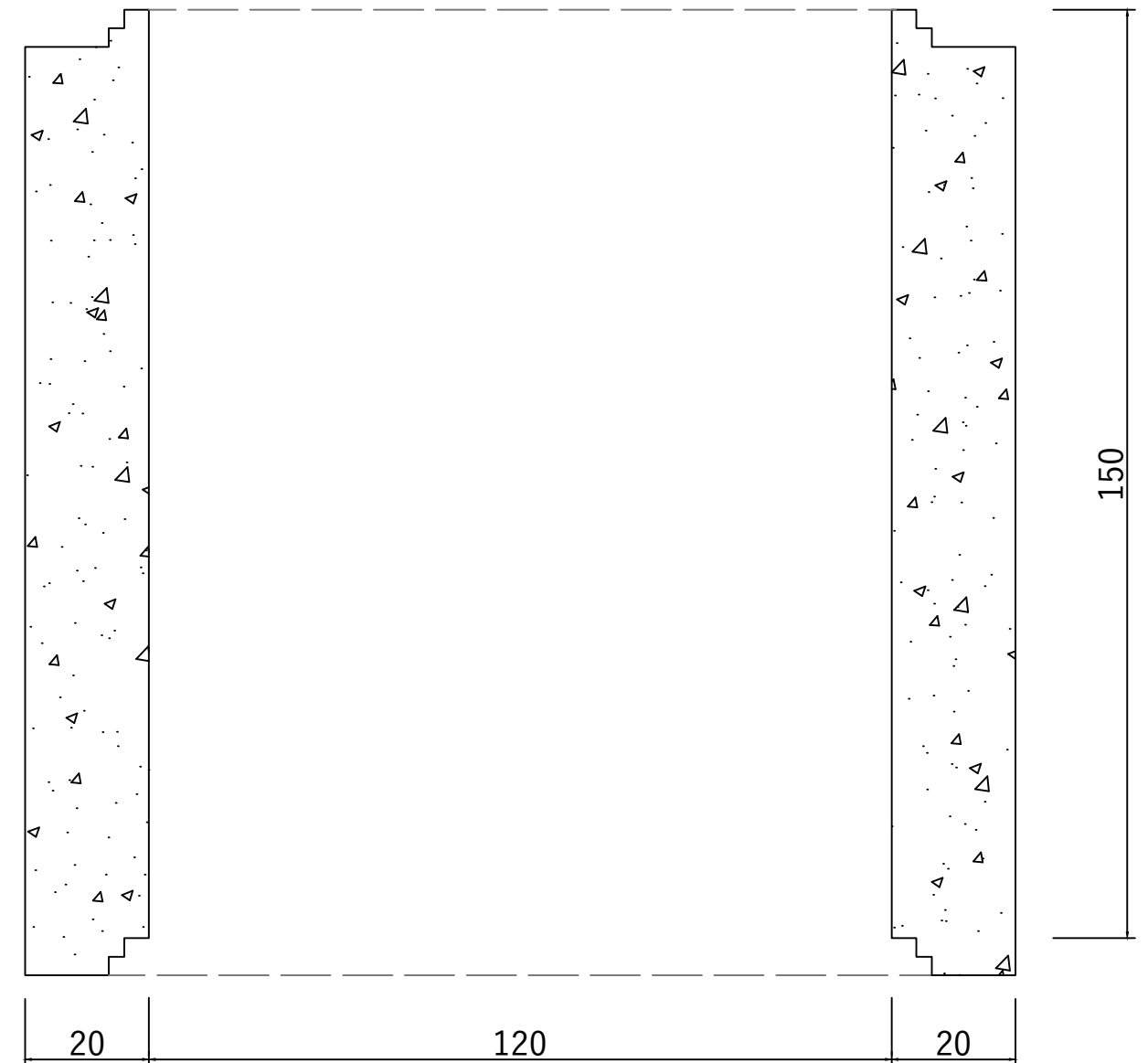
Sectiune Inel camin DN1200 H1500 G200
