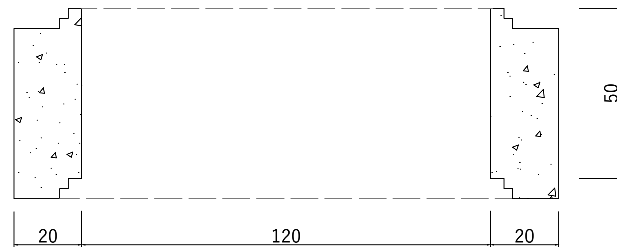
Sectiune Inel camin DN1200 H500 G200
