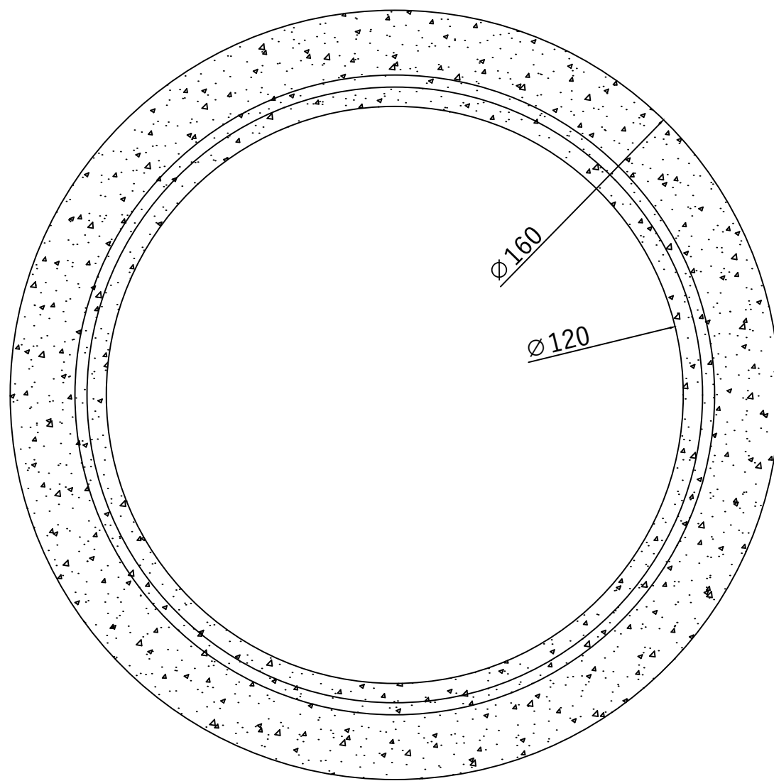
Vedere in plan Inel camin DN1200 H750 G200
