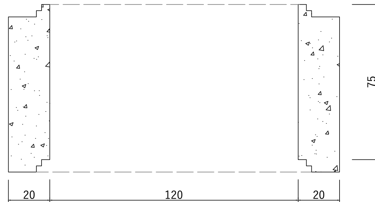
Sectiune Inel camin DN1200 H750 G200
