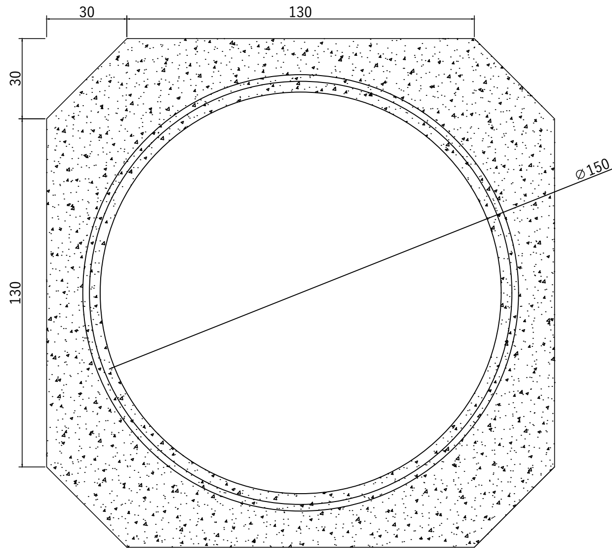
Vedere in plan Inel camin DN1500 H500 G200
