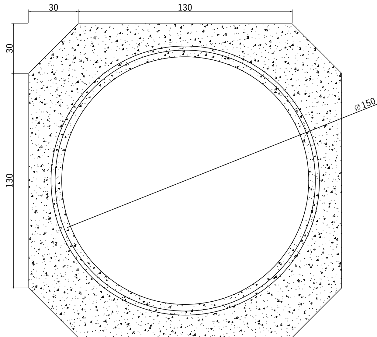
Vedere in plan Inel camin DN1500 H750 G200
