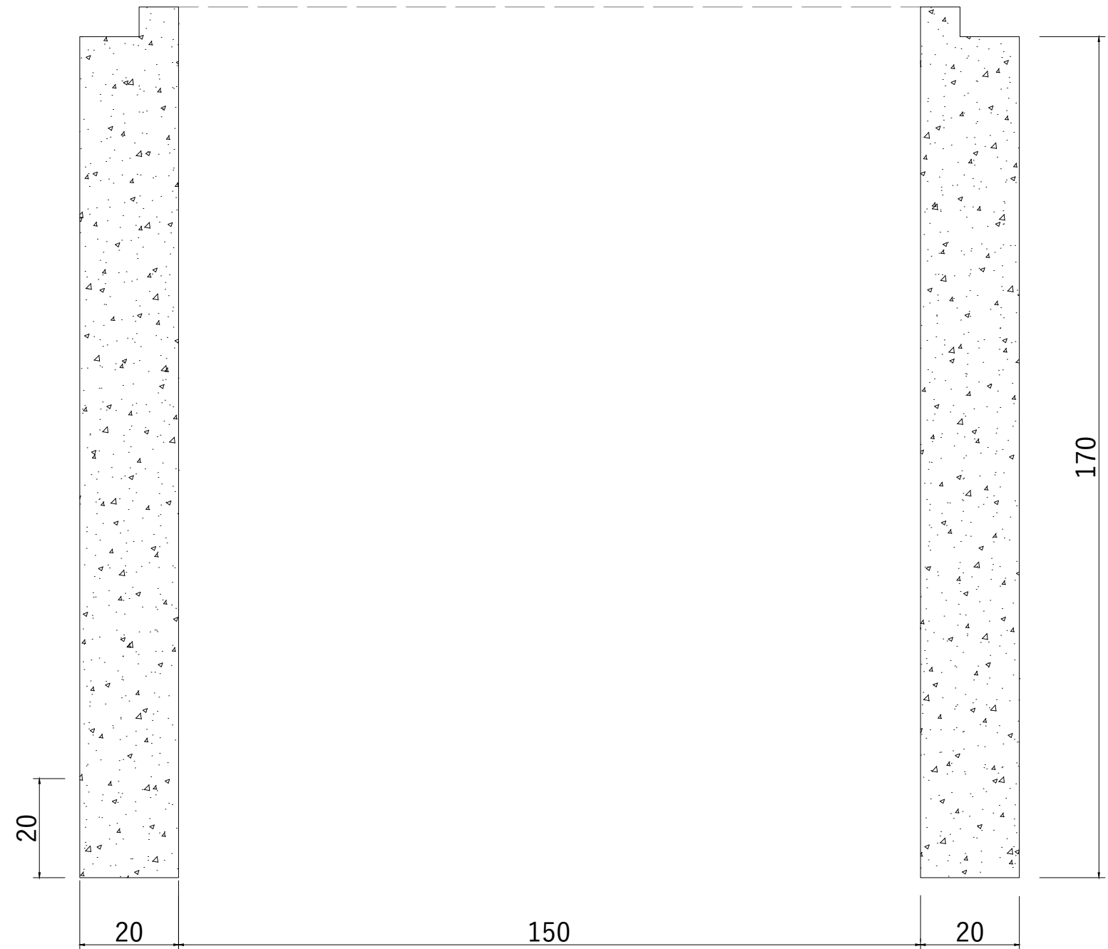
Sectiune Inel camin DN1500 H1700 G200
