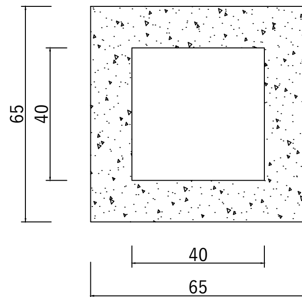
Vedere in plan Placa acoperire 650x650mm
