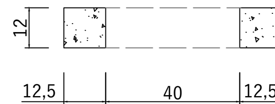
Sectiune Placa acoperire 650x650mm
