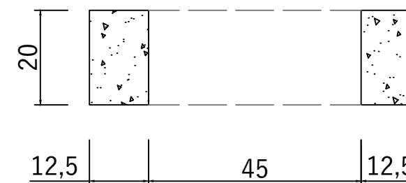
Sectiune Placa acoperire 700x700mm
