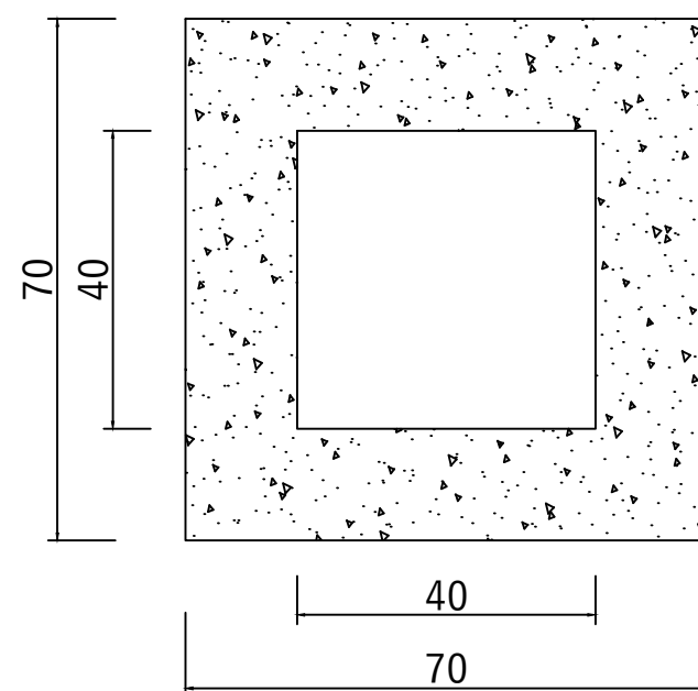
Vedere in plan Placa acoperire 700x700mm
