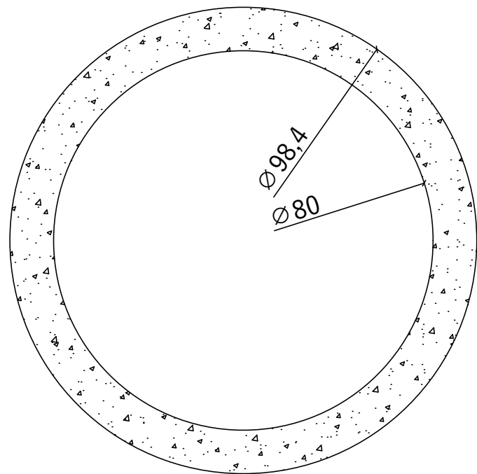
Vedere in plan Tub beton Ø 800mm
