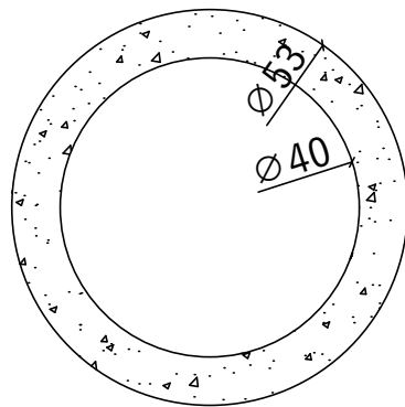
Vedere in plan Tub beton Ø 400mm
